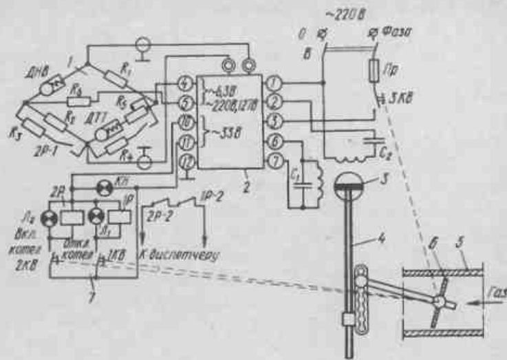
Рис.104. Принципиальная схема регулятора расхода газа РГА
