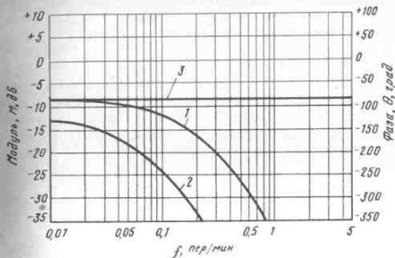
Рис.9. Логарифмические характеристики терморегулятора 1 - амплитудная (ЛАХ); 2 - фазовая (ЛФХ); 3 - усиление регулятора
