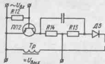
Рис. 47. Схема фазочувствительного выпрямителя ПТР-2
