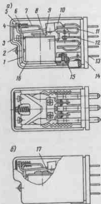
Рис. 76. Общий вид реле РПУ-0 а - для постоянного тока; б - для переменного тока
