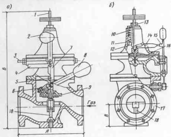
Рис. 25. Предохранительный запорный клапан а - вид сбоку со стороны ударника; б - вид со стороны выходного отверстия
