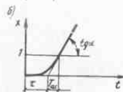
Рис. 5. Динамические свойства объектов а — статического; б — астатического
