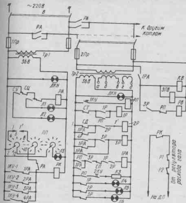
Рис.103. Принципиальная электрическая схема автоматики безопасности АГОК-66 В, 1В - выключатели; Tr - предохранитель; ЛКН - лампа контроля напряжения; СУ - сигнализатор уровня; СЦ - сигнализатор циркуляции; ПП - переключатель положений; РА - реле аварии; РК - реле контроля; РП - реле пуска; СТ - сигнализатор тяги; СД - сигнализатор давления; СП - сигнализатор перегрева; КЗ - катушка зажигания; КВ - контрольный вентиль; ЗПВ - запально-продувочный вентиль; РВ - рабочий вентиль; КУ - кнопка управления; Tr - трансформатор; Л1 - Л6 - лампы
