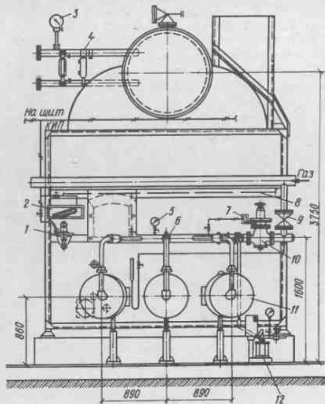
Рис. 109. Фронтальный вид котла ДКВР с автоматикой "Кристалл"
