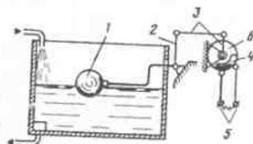
Рис.61. Схема поплавкового сигнализатора уровня СУ-3
