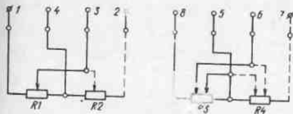
Рис. 86. Принципиальная электрическая схема соединения реостатов обратной связи блока реостатных датчиков БДР-1
