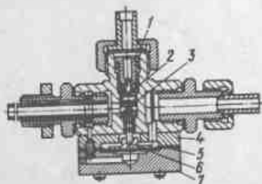
Рис. 23. Стабилизатор перепада давлений 1 - седло; 2 - пружина; 3 - клапан; 4 - корпус; 5 - мембрана; 6 - жесткий центр мембраны; 7 - крышка
