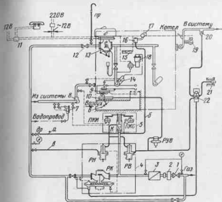
Рис.113. Схема пневмомеханической автоматики ПМА
