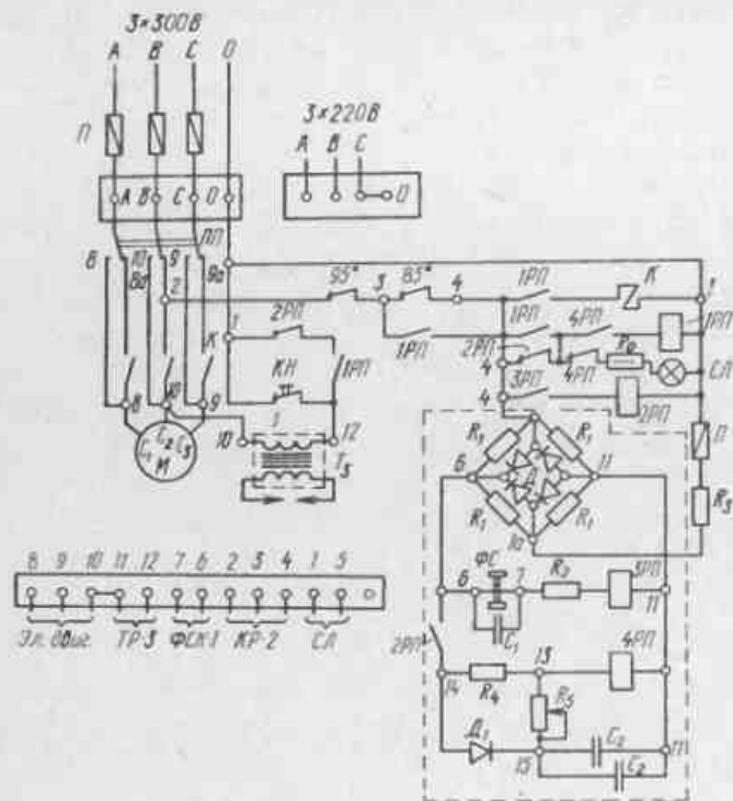
Рис.123. Принципиальная электрическая схема автоматизации механической форсунки
