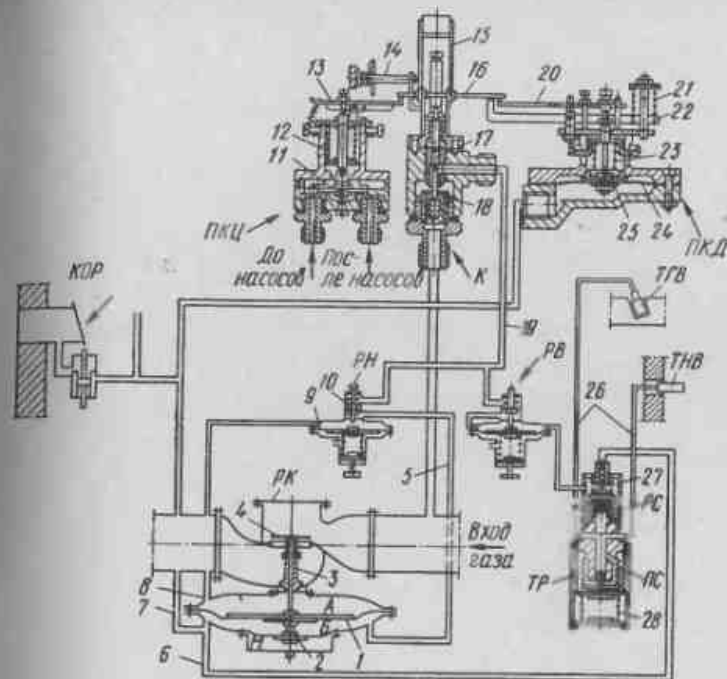
Рис.114. Приборы котловой автоматики безопасности ПМА
