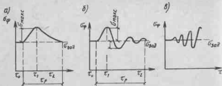
Рис. 6. Динамические характеристики процессов регулирования а - устойчивого апериодического процесса; б - устойчивого колебательного процесса; в - неустойчивого процесса
