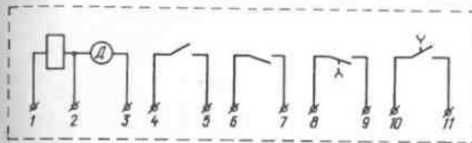
Рис. 79. Принципиальная схема реле времени РВ-4
