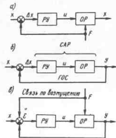
Рис.16. Блок-схемы САР
