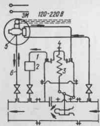
Рис.95. Схема работы регулятора давления с прибором телеуправления
