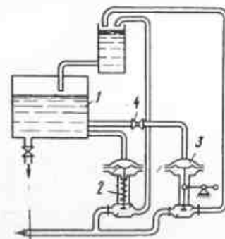
Рис.15. Схема изодромного регулятора
