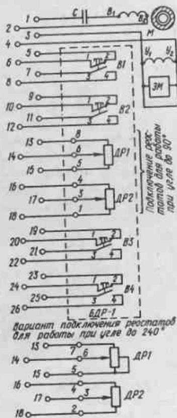
Рис. 87. Принципиальная электрическая схема исполнительных механизмов МЭО-1,6/40 и МЭО-4/100
