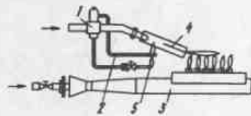
Рис. 64. Схема термоэлектрического контроля наличия пламени
