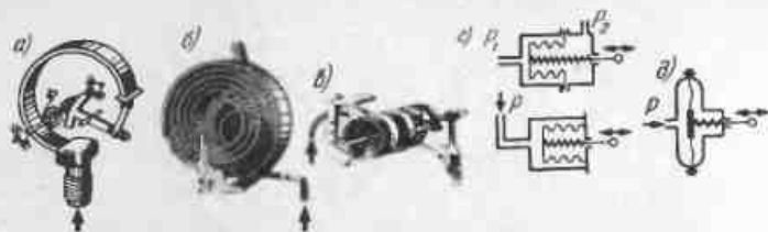
Рис. 28. Чувствительные элементы манометров а - трубчатая пружина; б - спиральная пружина; в - геликоидальная пружина; г - сильфоны внутреннего и внешнего действия среды; д - плоская мембрана
