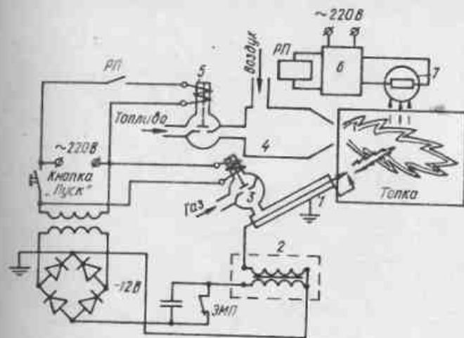
Рис. 69. Принципиальная схема запально-защитного устройства ЗЗУ
