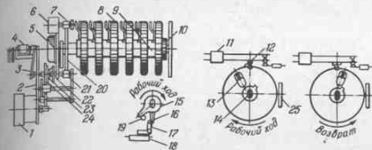
Рис.80. Кинематическая схема программного реле времени ВС-10
