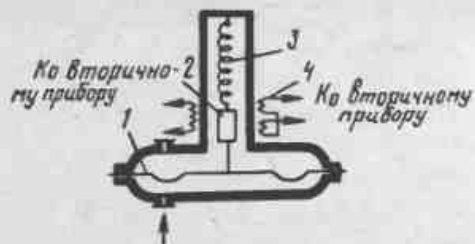
Рис.34. Принципиальная схема дифманометра ДМИ
