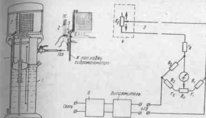
Рис. 88. Параметрическое устройство телеизмерения с реостатным датчиком
