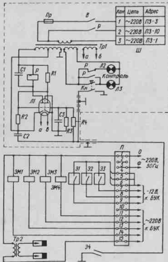
Рис. 134. Схема блока горения газообразного топлива
