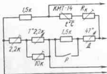
Рис.55. Схема подключения компенсирующего сопротивления в измерительный мост ПТР
