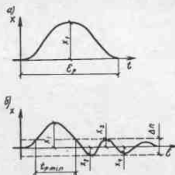
Рис.18. Типовые оптимальные переходные процессы при регулировании астатических объектов а — граничный аperiodический; б — с оптимальным временем регулирования
