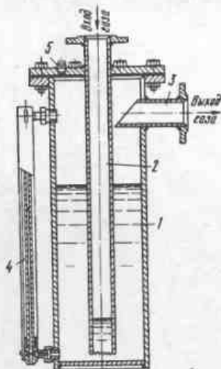
Рис.27. Гидравлический предохранительный затвор
