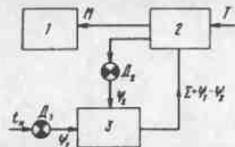
Рис. 2. Структурная схема регулирования теплопроизводительности котла
