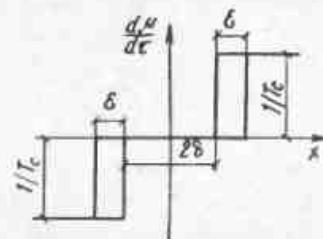
Рис.13. Характеристика регулятора постоянной скорости
