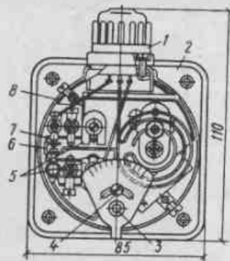
Рис. 39. Датчик-реле температуры ДТКМ
