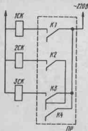
Рис. 140. Схема коммутации контактов для многоступенчатого регулирования 1СК – 3СК – электромагнитные клапаны; К1 – К4 – контакты позиционного регулятора; ПР – позиционный регулятор
