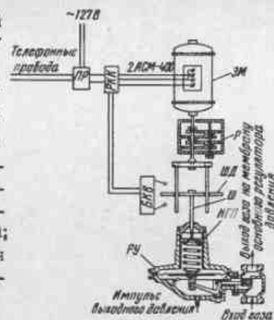
Рис. 94. Исполнительный механизм с "пилотом" РЖГД
