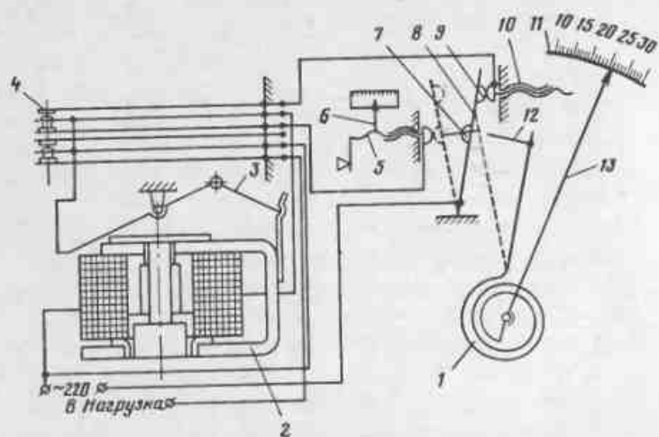
Рис.40. Схема камерного биметаллического датчика-реле температуры ТБ-Э2К
