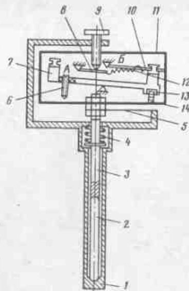
Рис.42. Схема дилатометрического контактного устройства ТУДЭ с нормально замкнутыми контактами
