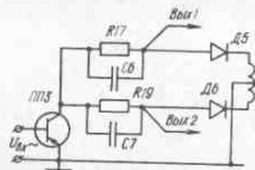
Рис. 51. Фазочувствительный выпрямитель ПТР-3
