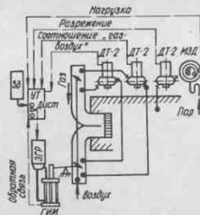
Рис.107. Принципиальная схема электрогидравлической системы автоматики "Кристалл"
