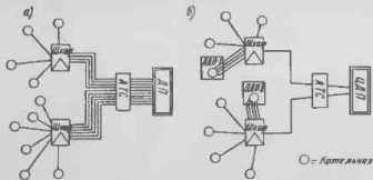
Рис. 99. Структурные схемы систем диспетчеризации котельных а — одноступенчатой; б — двухступенчатой
