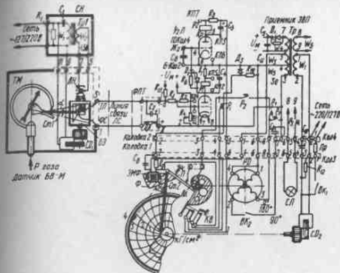
Рис. 93. Принципиальная схема время-импульсного устройства телеизмерения ТВ-1
