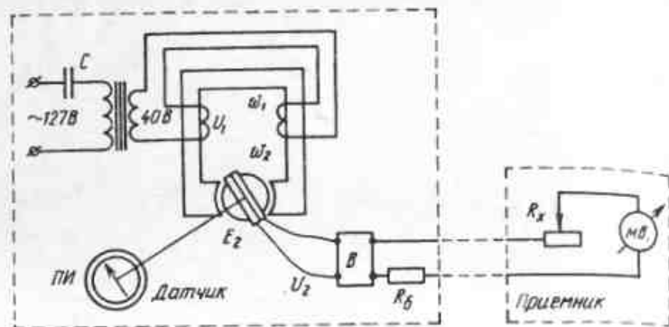
Рис.89. Принципиальная схема устройства телеизмерения с индукционным рамочным датчиком
