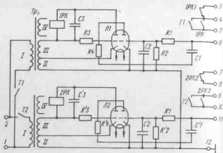
Рис. 73. Принципиальная схема автомата контроля пламени АКП-П
