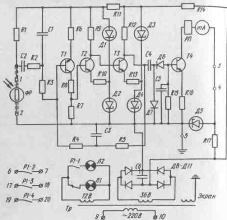
Рис. 72. Принципиальная схема управляющего прибора 33У
