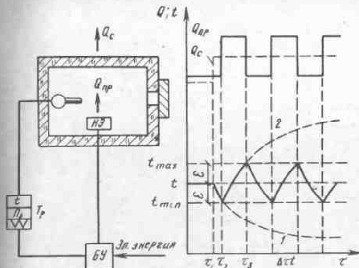
Рис. 11. Двухпозиционное регулирование температуры
