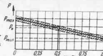
Рис.10. Статическая характеристика регулятора давления
