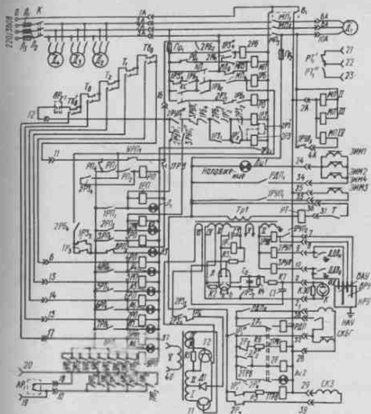
Рис. 117. Принципиальная электрическая схема системы автоматизации АМКО микрокотлов К - выключатель пакетный; ТВ в - предельный терморегулятор горячей воды; Т т - предельный терморегулятор температуры мазута; Т - датчик разрежения; Т в - датчик давления воздуха; ТВ г - контакт общекотельного регулятора ПРП; АР 2-7 - контакты сигнализации автоматического ввода резерва циркуляционного насоса; Д 1 - электродвигатель вентилятора; Д 2 - электродвигатель топливного насоса; Д 3 - электродвигатель водяного насоса; Д 4 - электродвигатель дымососа; ДДВ н , ДДВ в - реле давления воды РД-12; КЭО - контрольный электрод газового пламени; ФД - фотодатчик пламени жидкого топлива; Л - электронная лампа 6Н6П (остальные обозначения в тексте)
