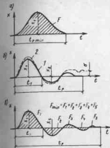
Рис.17. Типовые оптимальные переходные процессы при регулировании статических объектов
