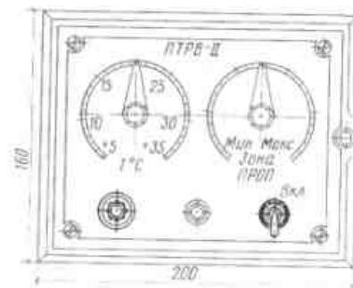
Рис. 57. Общий вид панели ПТРВ.
