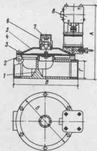
Рис. 82. Общий вид конструкции клапанов КГ-20, КГ-40, КГ-70
