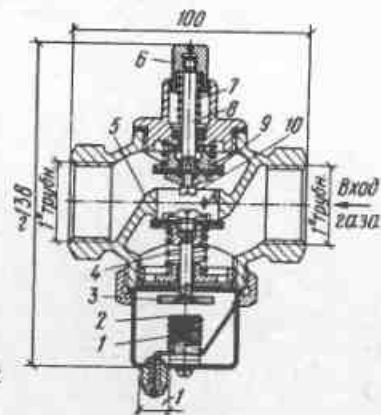
Рис. 65. Электромагнитный клапан
