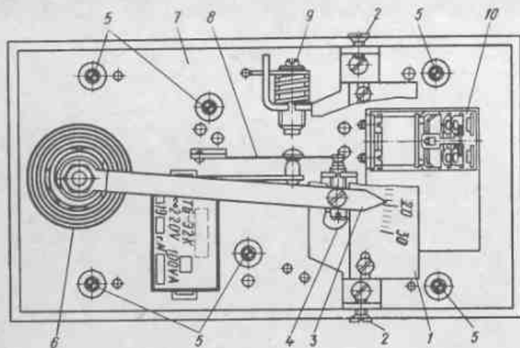
Рис.41. Общий вид датчика-реле температуры ТБ-32К (со снятой крышкой)
