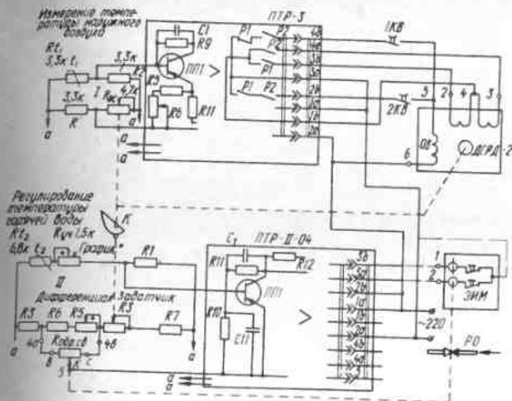
Рис. 59. Схема полупроводникового регулятора температуры ПТР-НК с автокоррекцией по наружной температуре
