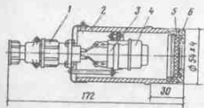
Рис. 71. Общий вид фотодатчика
