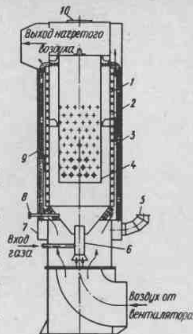
Рис. 138. Принципиальная схема газоздушного калорифера К-350
