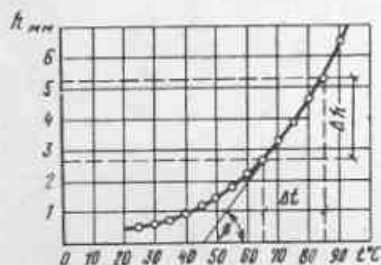
Рис. 4. Статистическая характеристика терморегулятора
