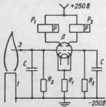
Рис. 67. Принципиальная схема прибора контроля пламени института Ленгипроинжпроект Э - электрод; Г - горелка; Р1 - Р2 - обмотки поляризованного реле; Л - радиолампа 6Н2И; С - конденсатор; 1 - 3 - сопротивления
