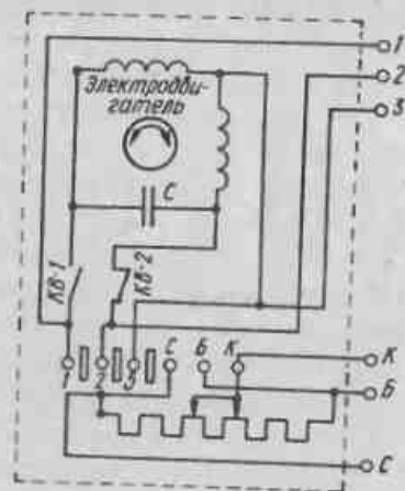
Рис. 84. Принципиальная электрическая схема ПР-М
