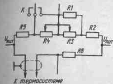
Рис. 46. Элемент схемы усилителя ПТР-2
