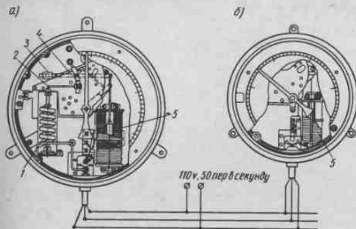
Рис.32. Комплект электроиндукционного манометра МУЭ
