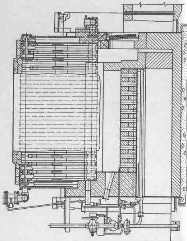
Рис. 111. Продольный разрез секционного котла "Универсал-6" с форкамерной горелкой и автоматикой ПМА
