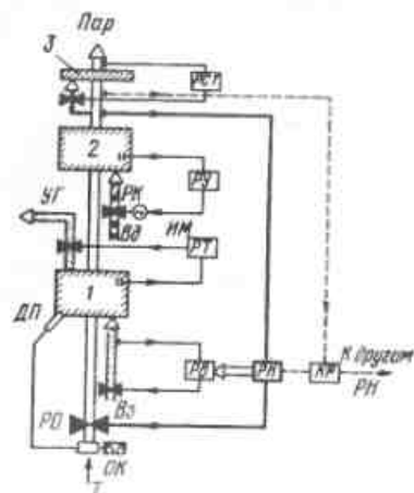
Рис. 3. Схема регулирования технологических процессов в котельной установке
