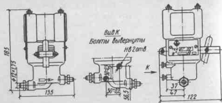
Рис. 81. Общий вид и габаритные размеры электромагнитного клапана КГ-10
