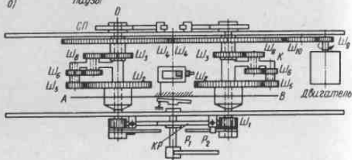
Рис. 92. Схема приемного прибора время-импульсного устройства
