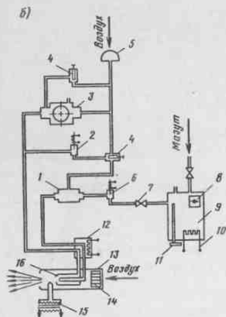
Рис.126. Мазутная форсунка МАФ-66
