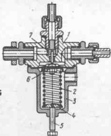
Рис. 24. Ускорительный клапан 1 - корпус; 2 - мембрана; 3 - крышка; 4 - клапан; 5 - регулировочный винт; 6 - тарелка пружины; 7 - шток; 8 - пружина
