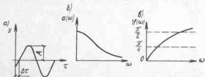
Рис. 7. Частотные характеристики объекта с самовыравниванием
