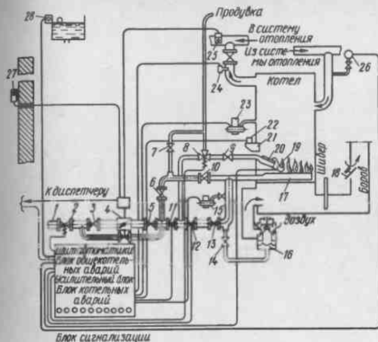
Рис. 102. Принципиальная технологическая схема автоматизации газового отопительного котла по системе АГОК-66
