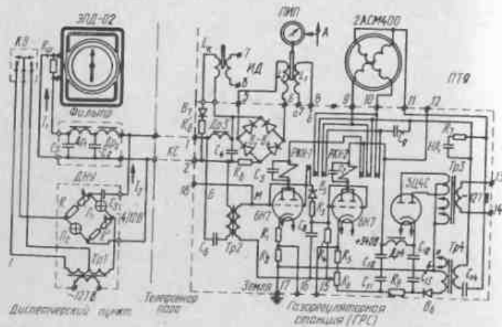
Рис.97. Принципиальная схема устройства непрерывного телеизмерения и телеуправления по одной паре проводов
