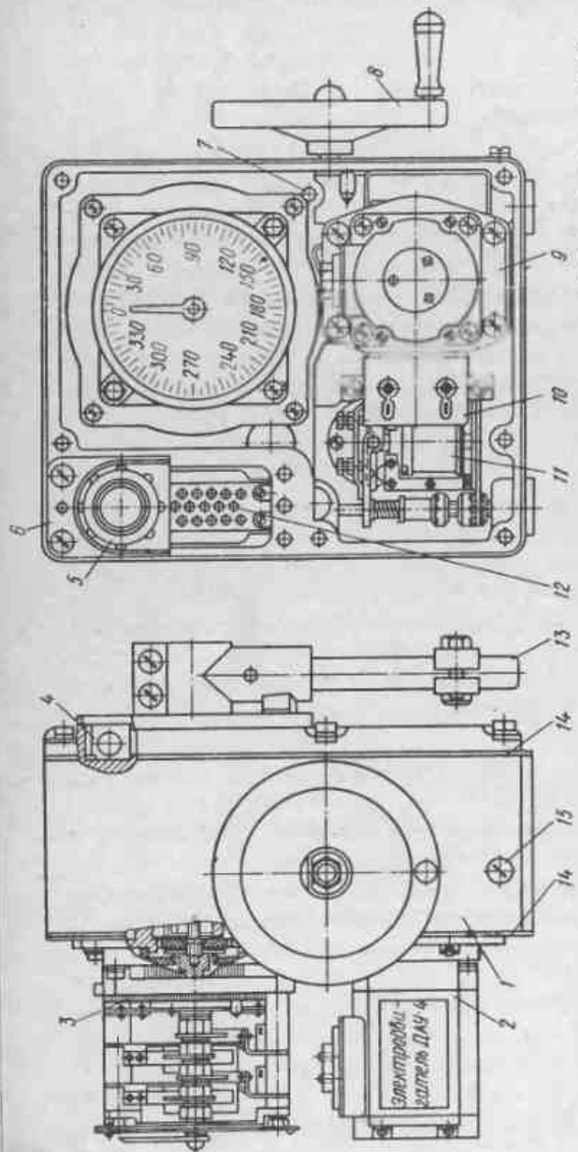
Рис. 85. Конструкция электрических исполнительных механизмов МЭО-1,6/40 и МЭО-4/100
