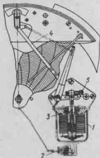
Рис.31. Схема манометра МС
