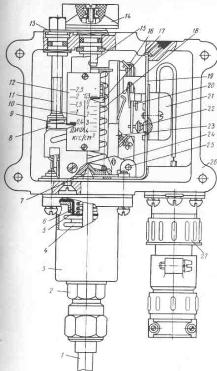
Рис.37. Конструкция датчика - реле давления РД
