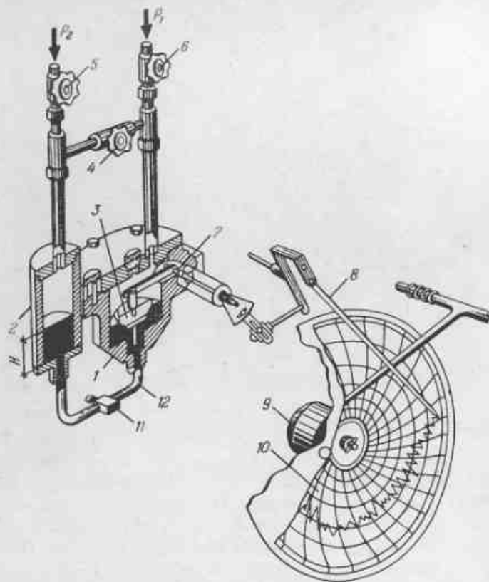
Рис.33. Схема расходомера ДП
