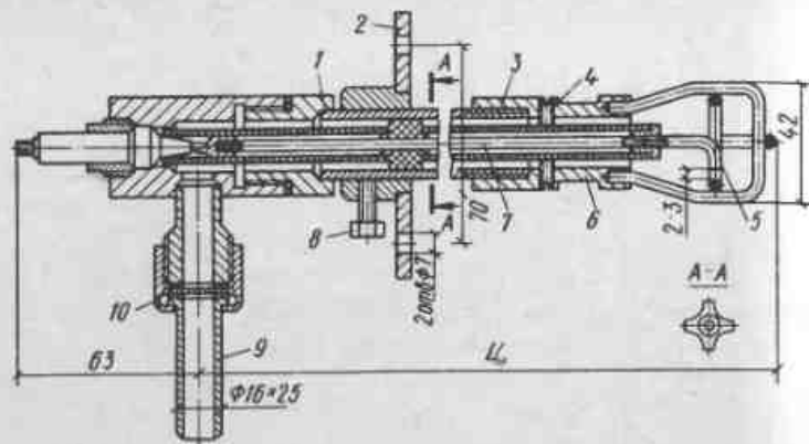
Рис. 70. Конструкция электрозапальника
