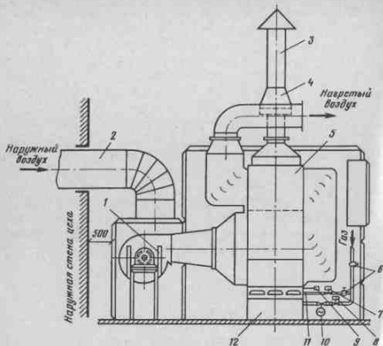
Рис.135. Схема газовой воздушного отопительно-вентиляционного агрегата
