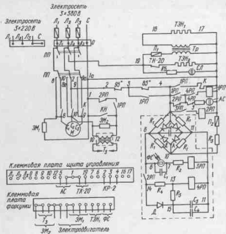
Рис.127. Принципиальная электрическая схема автоматического управления работой форсунки МАФ-66
