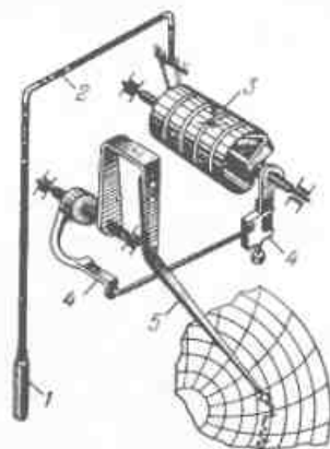
Рис.38. Схема манометрического термометра
