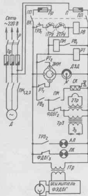
Рис. 125. Принципиальная схема автоматизации отопительного водогрейного котла с механической форсункой НИИСантехники
