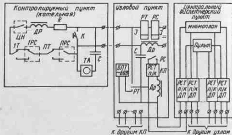
Рис.100. Принципиальная схема диспетчеризации отопительных котельных
