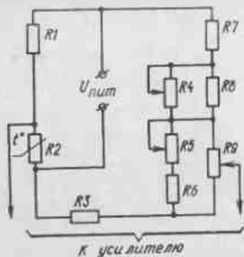
Рис. 53. Схема измерительного моста ПТР-П
