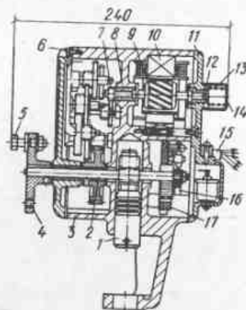
Рис.83. Конструкция моторного электрического исполнительного механизма ПР-М
