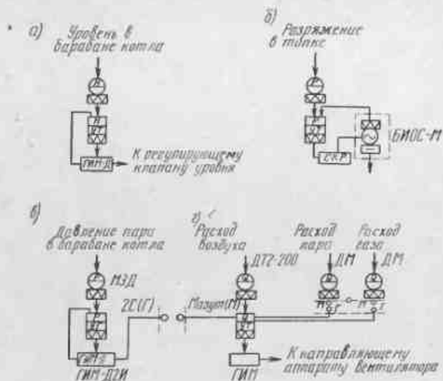
Рис. 108. Схема регуляторов в системе автоматизации "Кристалл" а - регулятор уровня; б - регулятор разрежения; в - регулятор топлива; г - регулятор воздуха
