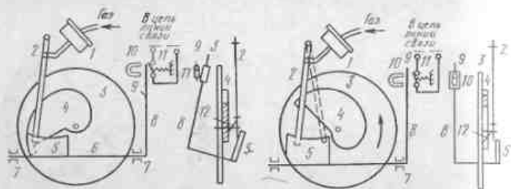
Рис. 91. Кинематическая схема время-импульсного датчика
