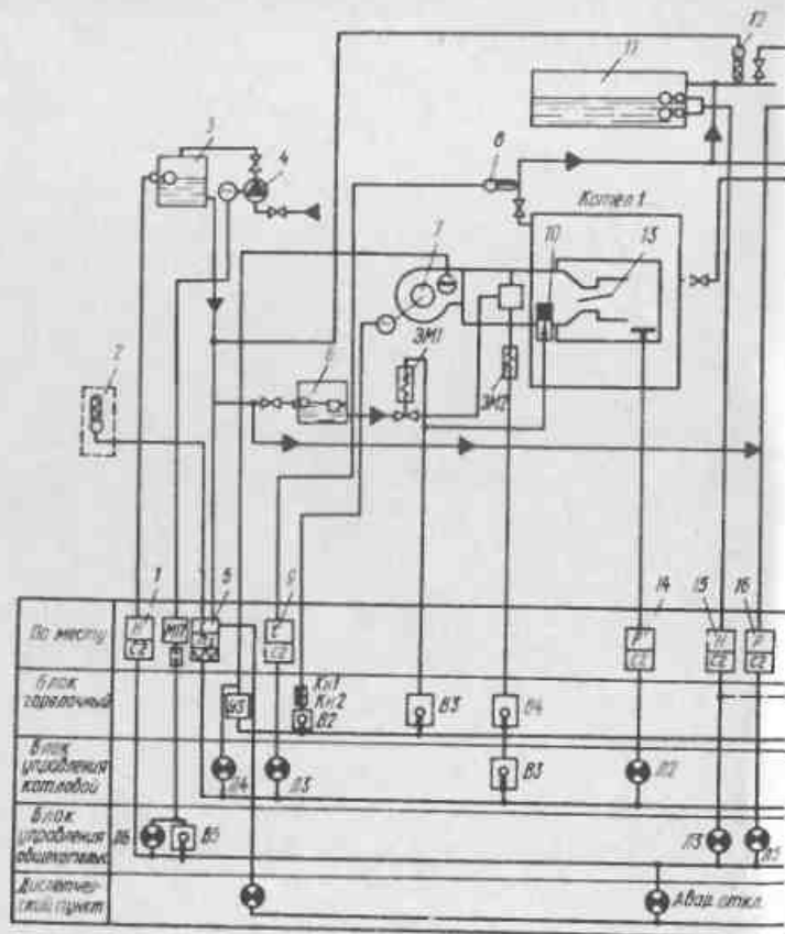
Рис. 132. Общая функциональная электрическая схема автоматики "Пламя"
