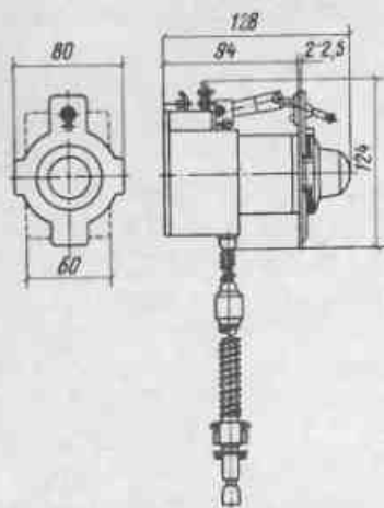
Рис. 44. Общий вид терморегулятора ТР5-К
