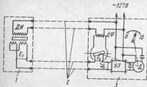
Рис.35. Схема дистанционной передачи измерений на вторичный прибор ВФ 1 - дифманометр ДМИ; 2 - линии связи; 3 - вторичный прибор ВФ
