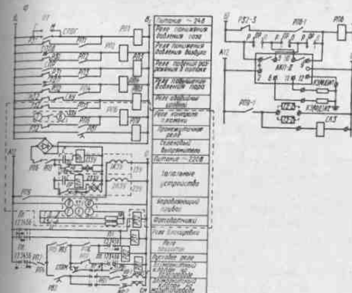
Рис.110. Принципиальная схема автоматики безопасности "Кристалл". а - в комплекте с ЗЗУ; б - в комплекте с АКП-П
