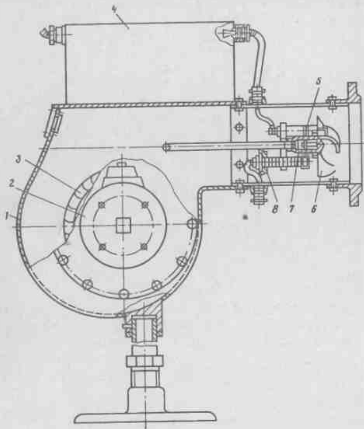
Рис.124. Механическая форсунка НИИСантехники 1 - корпус; 2 - электродвигатель; 3 - вентилятор; 4 - трансформатор зажигания; 5 - электроды зажигания; 6 - завихритель; 7 - распылитель топлива; 8 - фотодатчик
