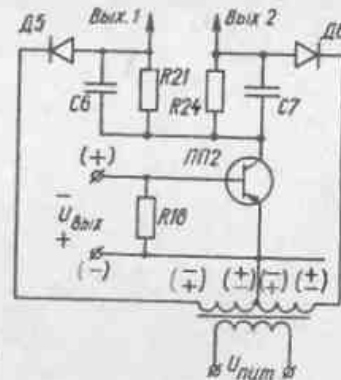
Рис. 54. Схема фазочувствительного выпрямителя ПТР-П
