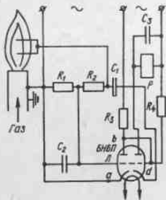
Рис. 66. Принципиальная электрическая схема прибора контроля пламени системы Ленпроменергогаз 1 - 4 - сопротивления; C1 - C3 - конденсаторы; Л - лампа 6W6P; P - реле
