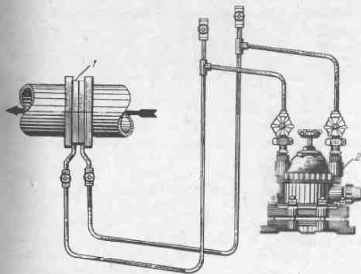
Рис.36. Схема присоединения дифманометра ДМИ к дроссельному органу
