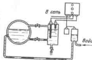
Рис.62. Принципиальная схема установки и контроля уровня воды в паровом котле посредством электронного двухпредельного сигнализатора уровня ЭСУ-2М
