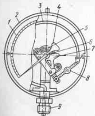
Рис. 29. Устройство показывающего манометра с одновитковой пружиной
