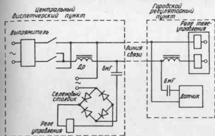
Рис.96. Схема измерения давления газа и телеуправления по одной паре проводов
