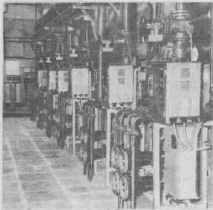
Рис.118. Общий вид котельной с котлами "ГАЗ-900", оборудованными системой автоматизации АМКО
