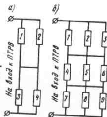
Рис. 58. Принципиальные схемы соединений датчиков ДПТРВ для усреднения командного импульса а - для четырех датчиков б - для девяти датчиков
