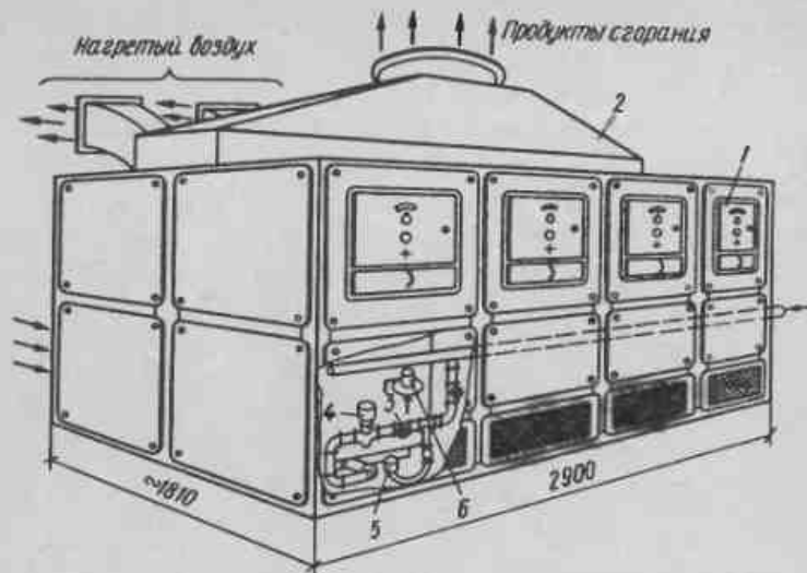
Рис.136. Общий вид газового отопительно-вентиляционного агрегата, состоящего из нескольких блоков
