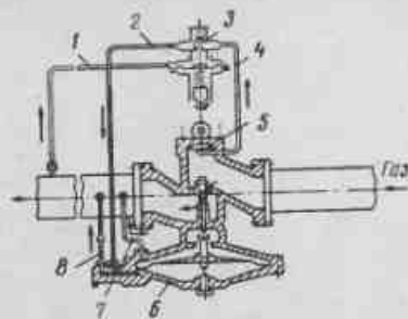
Рис.21. Схема регулятора давления РДУК-2-100
