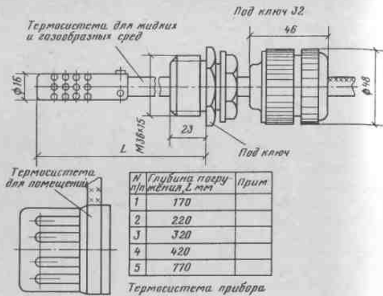
Рис. 48. Термосистемы полупроводниковых регуляторов температуры
