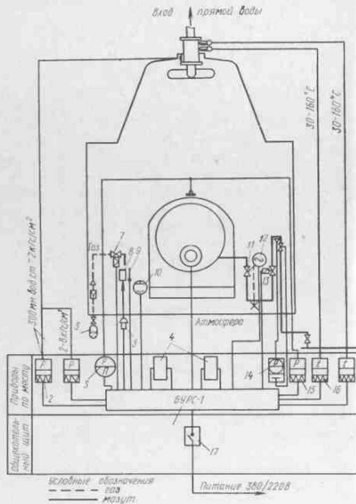
Рис.121. Функциональная схема автоматизации котла "Универсал-6М" на тяжелом жидком топливе 1 - блок БУРС-1; 2 - реле давления РД-12-01; 3 - тягонапормер ТНЖ; 4 - промежуточное реле РПУ-1; 5 - bobина зажигания Б-1; 6 - бал-
