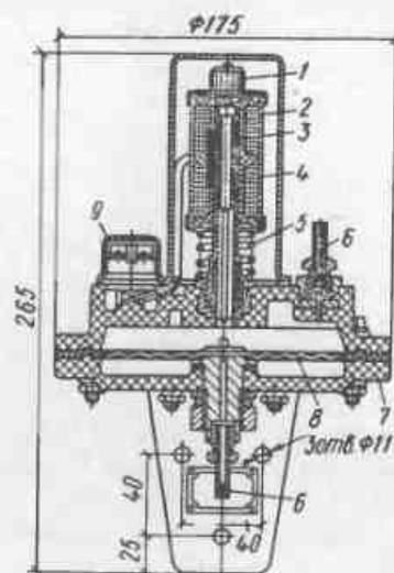
Рис. 75. Дифференциальный тягомер ДТ-2
