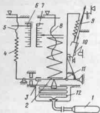
Рис.8. Схема манометрического термометра
