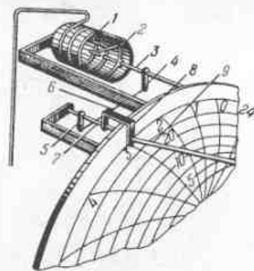
Рис. 30. Схема самопишущего манометра МГ с геликоидальной пружиной
