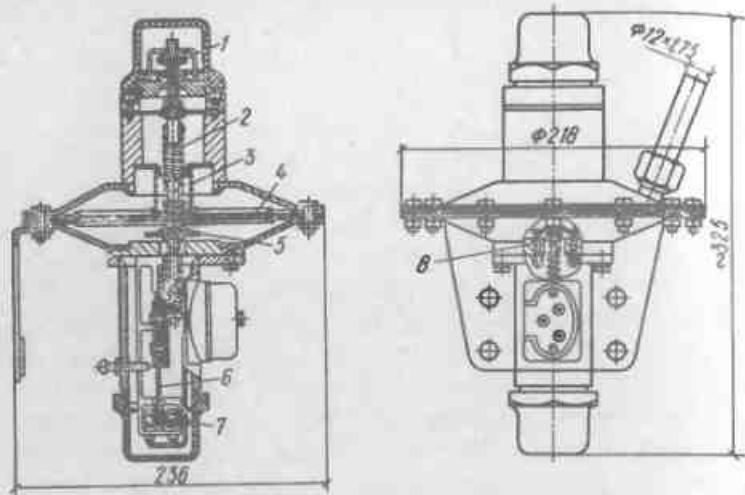
Рис. 74. Сигнализатор падения давления СПД-1
