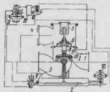
Рис.22. Схема унифицированного регулятора давления РДУК-2-М-100
