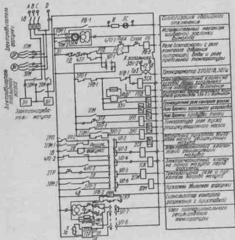
Рис.129. Принципиальная электрическая схема автоматического управления котлоагрегатом, оборудованным ротационной форсункой
