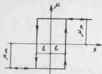
Рис.12. Характеристика двухпозиционного регулятора
