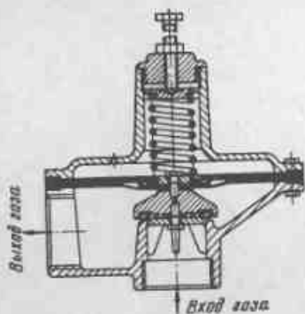
Рис.26. Пружинный сбросной клапан
