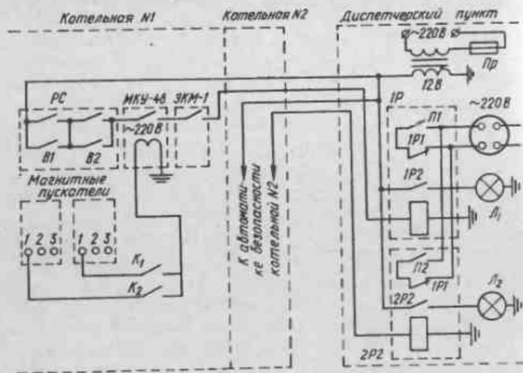
Рис.101. Система диспетчеризации котельных г. Днепропетровска
