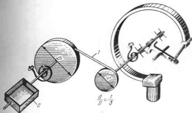
Рис.90. Кинематическая схема соединения рамок с осью манометра
