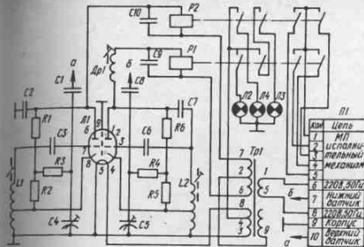
Рис. 63. Принципиальная электрическая схема прибора ЭСУ-2М
