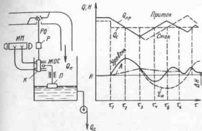
Рис.14. Регулирование уровня П-регулятором
