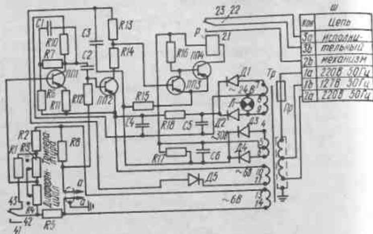
Рис. 45. Схема полупроводникового двухпозиционного регулятора температуры ПТР-2
