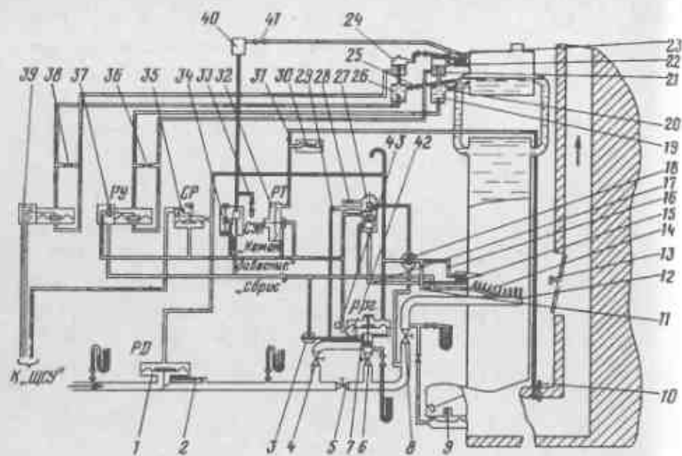
Рис.115. Принципиальная схема пневматической автоматики АГК-2П
